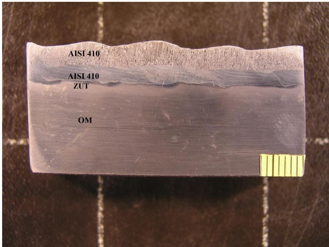
Slika 29 Makroizbrusak 1
