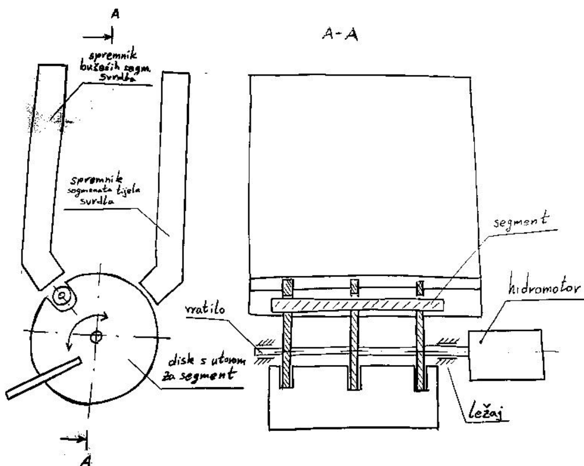
Slika 19. Prikaz koncepta 1
