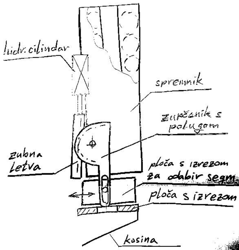
Slika 23. Prikaz koncepta 3
