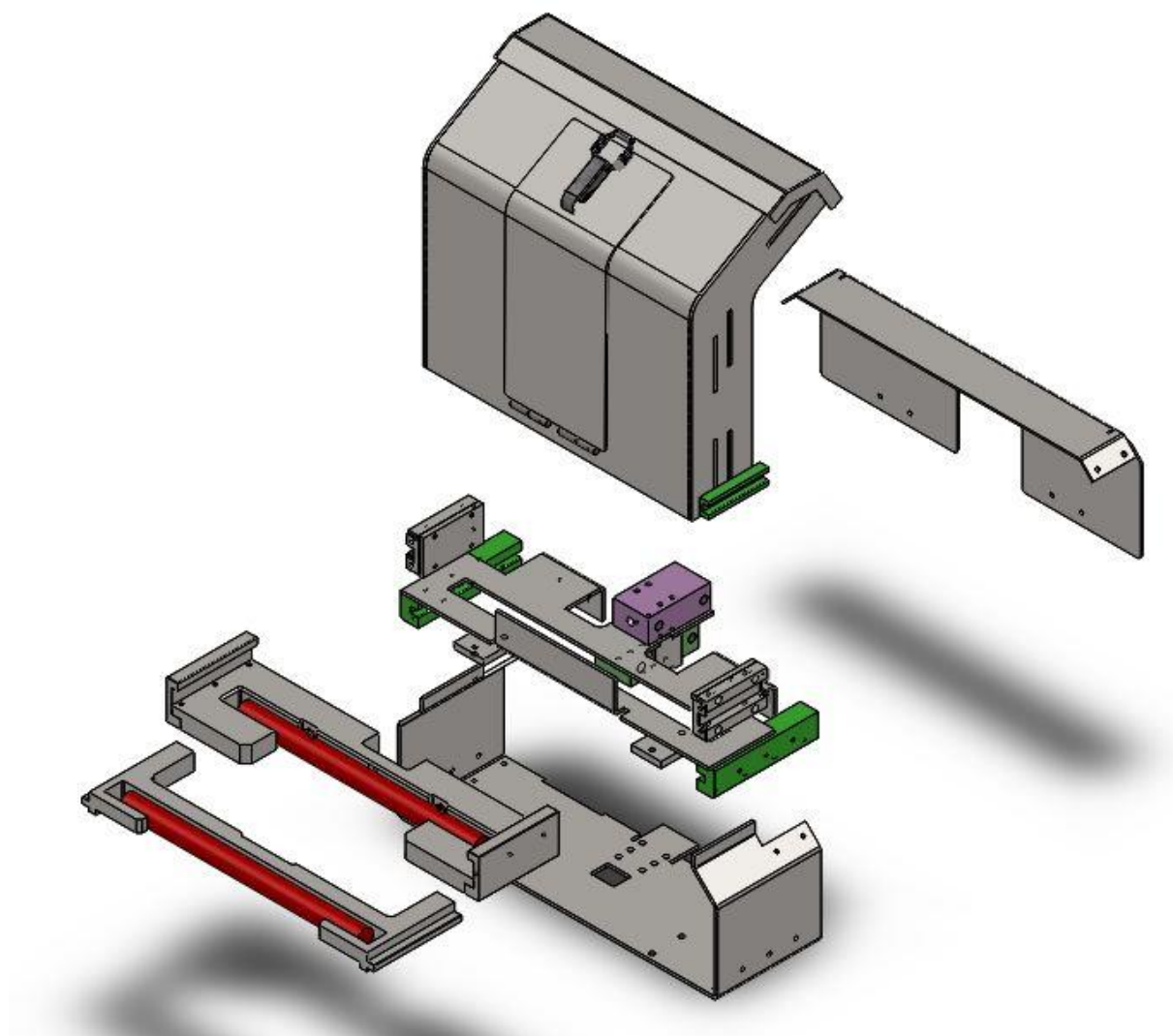
Slika 29. Eksplodirani prikaz stroja za dobavu segmentiranih svrdla
