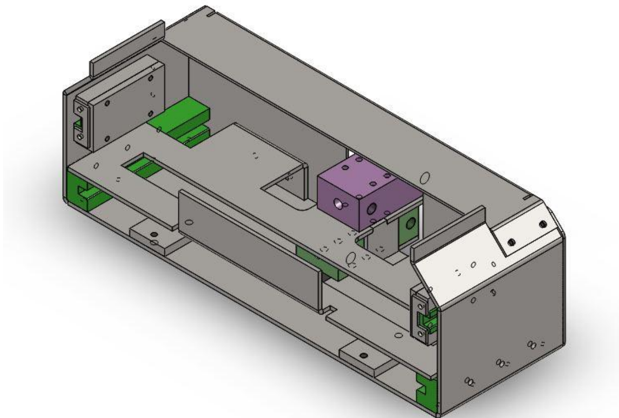
Slika 36. Nosač spremnika segmenata i hidrauličkih blok cilindara
