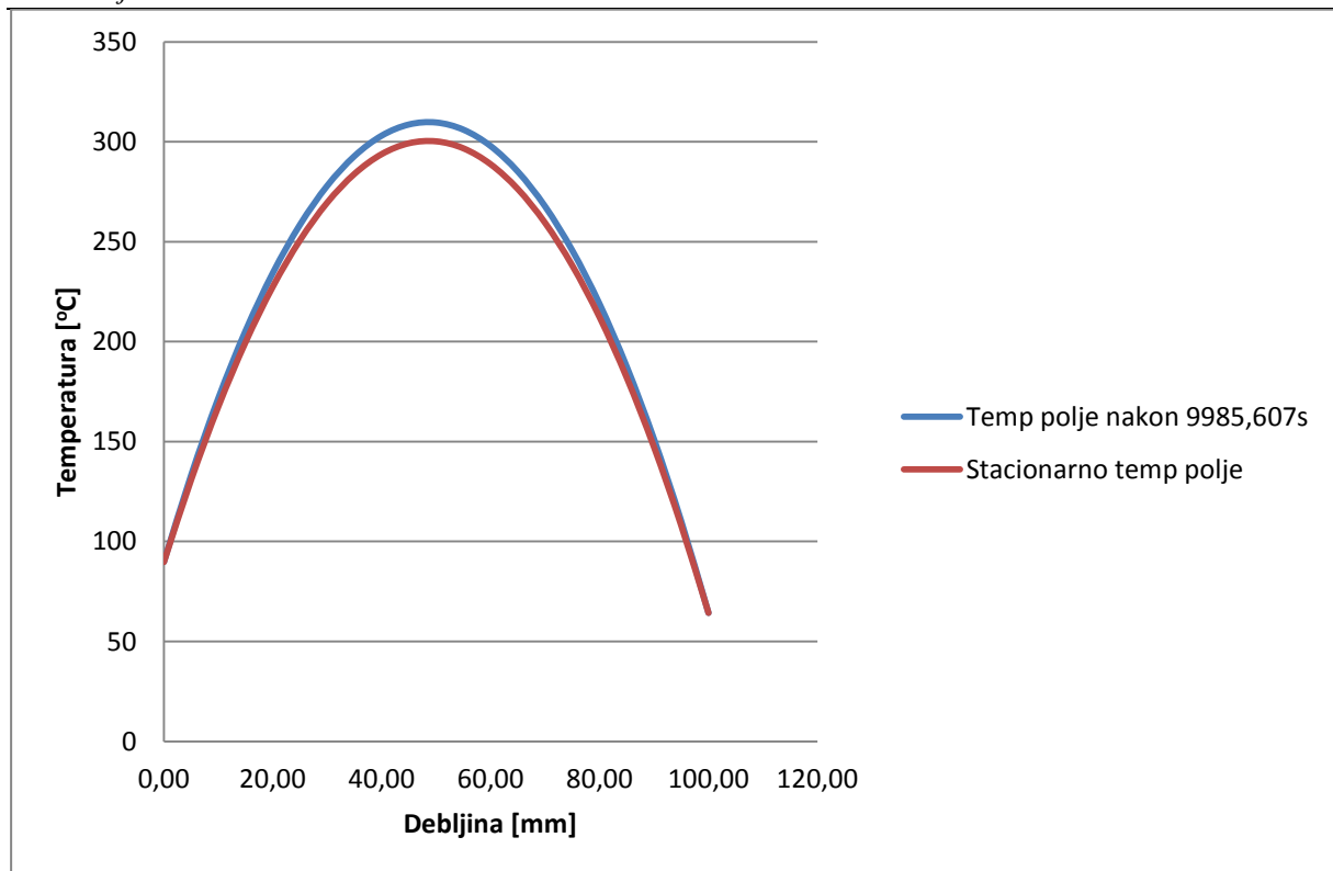
Slika 19. Aproksimacija temperaturnog polja u azbestu za \Phi_v = 20000 \text{ W/m}^3
