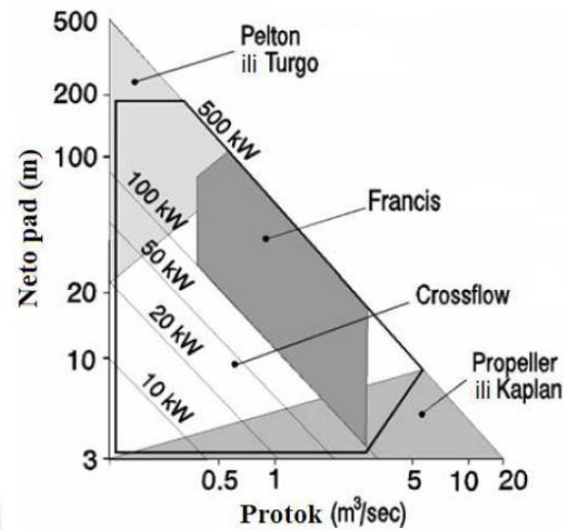
Slika 14. Dijagram za radna područja pojedinih turbina
