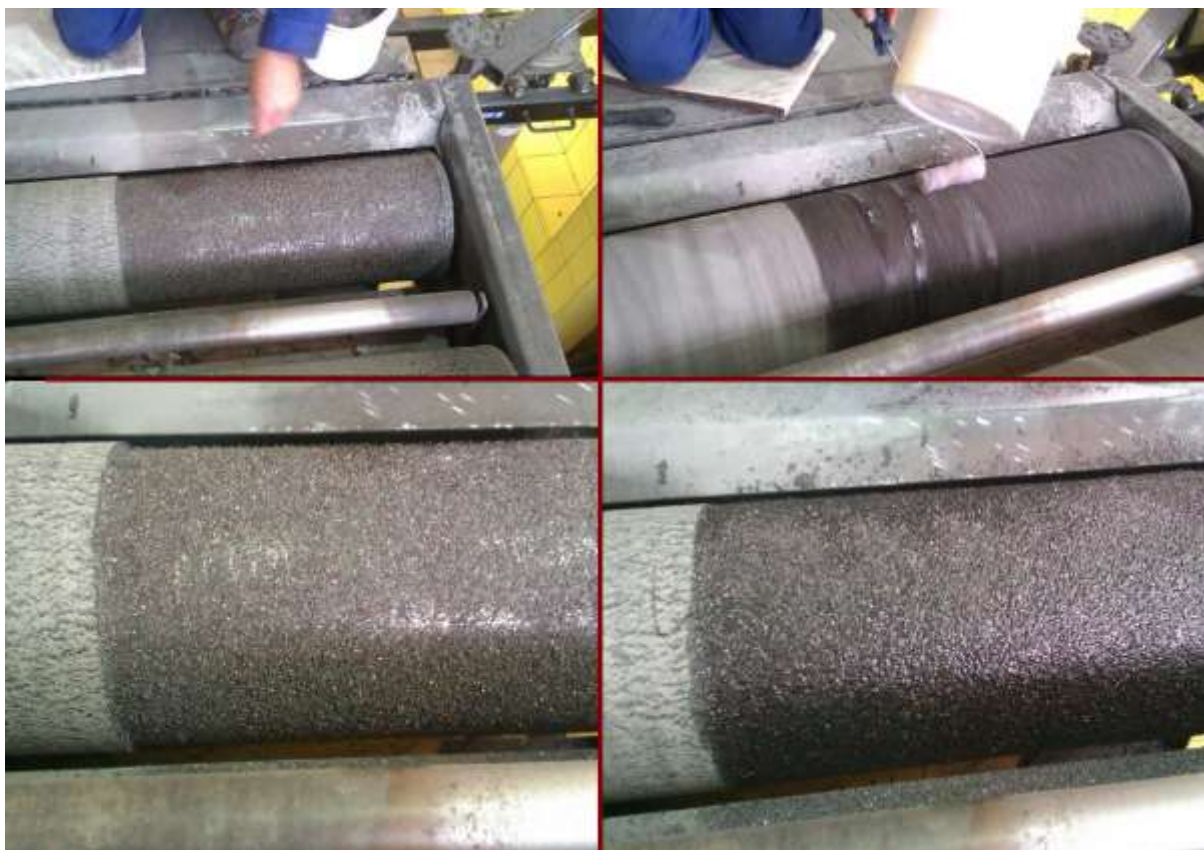
Slika 30. Postupak nanašanja čestica korunda i smole
