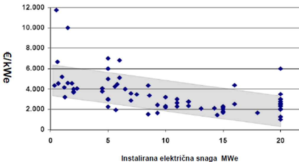
Slika 12. Specifični investicijski troškovi kogeneracijskih postrojenja područnog grijanja [28]
