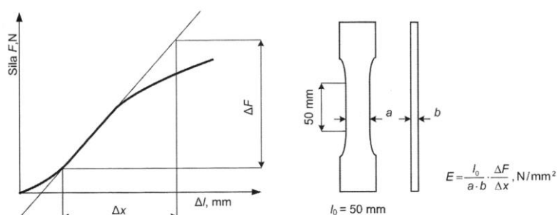
Slika 5.7. Postupak određivanja modula elastičnosti polimernih materijala [2]
