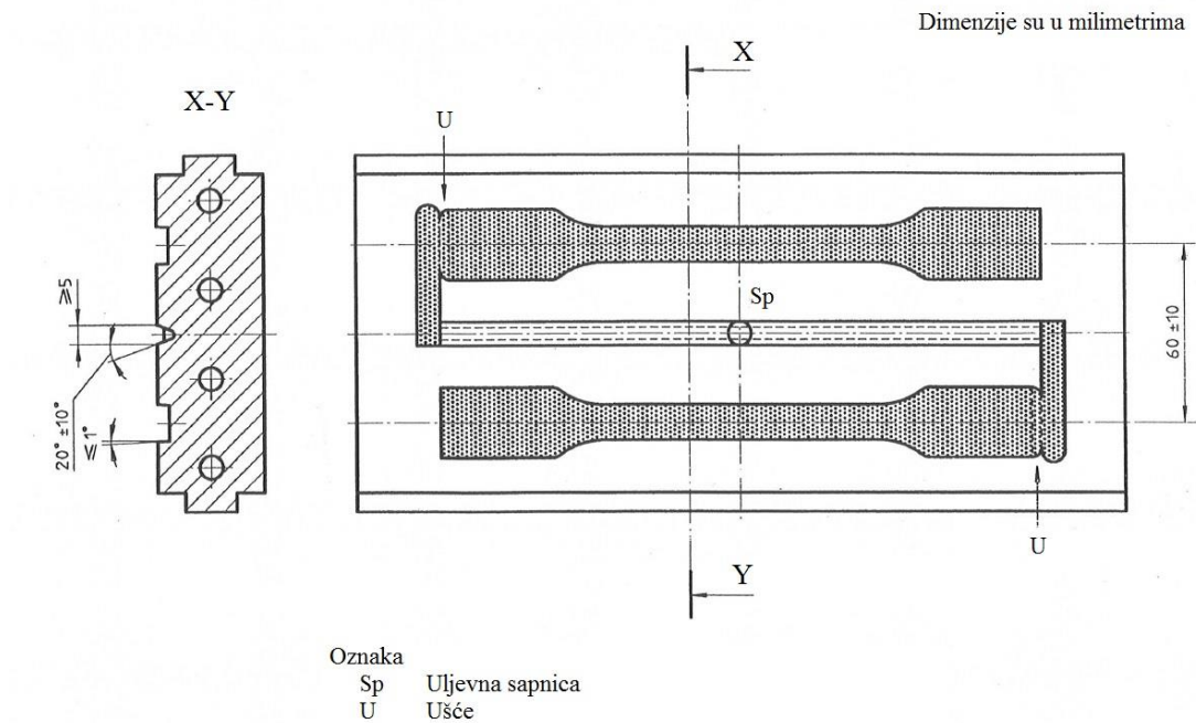
Slika 3.2. Kalupna ploča za ISO kalup tipa A [15]
