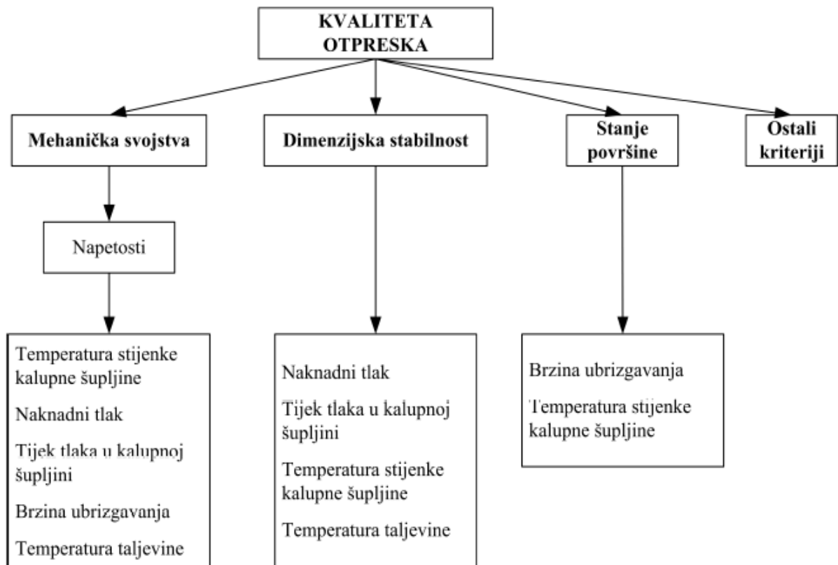
Slika 2.12. Kvaliteta otpreska u ovisnosti o parametrima preradbe [3,7]
