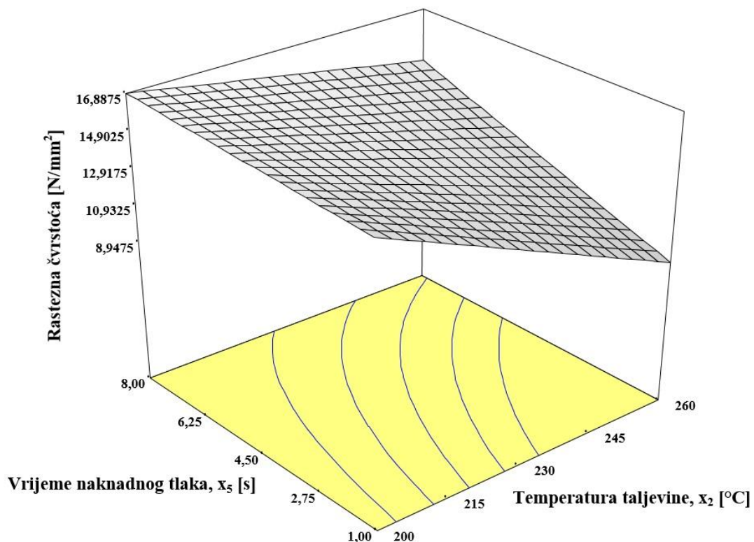
Slika 6.15. Ovisnost rastezne čvrstoće o temperaturi taljevine i vremenu naknadnog tlaka u pretpokusu
