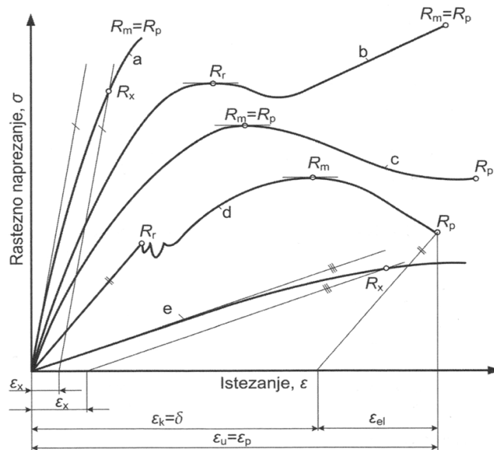
Slika 5.6. Vrste krivulja pri ispitivanju rastežanjem: a – sivi lijev ili PS, PMMA, UP; b – PE-LD; c - PA ili PE; d – niskouglični čelik; e – Al, Cu, PA [2]
