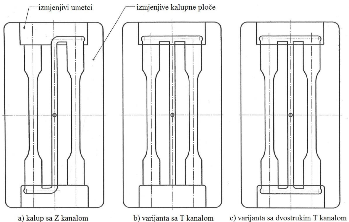
Slika 3.4. Različite konfiguracije umetaka [15]
