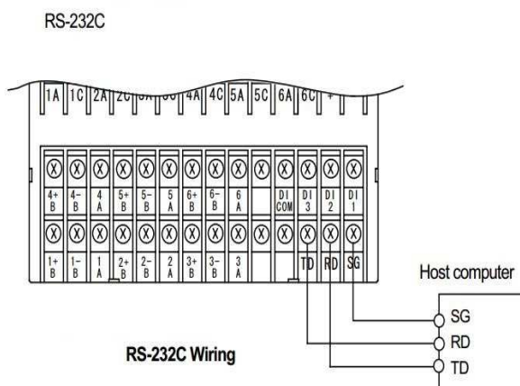
Slika 36. Shema spajanja računala s registratorom temperature
