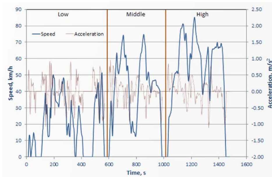
Slika 2.7. WLTP kategorija 2 [10]
