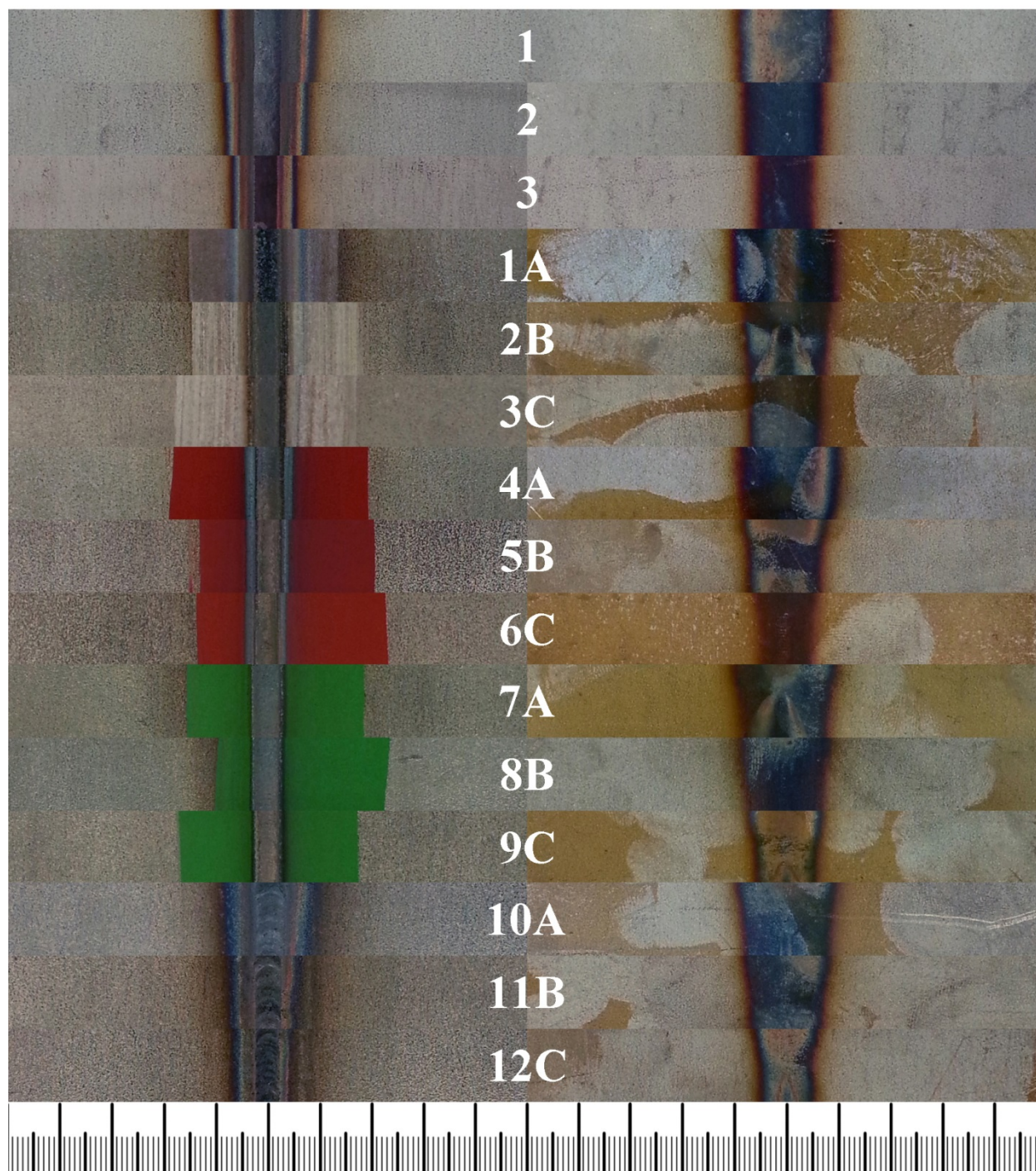
Slika 56. Izgled navara svih ispitnih uzoraka
