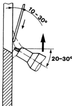
Slika 14. Ručno TIG zavarivanje odozdo prema gore [1]
