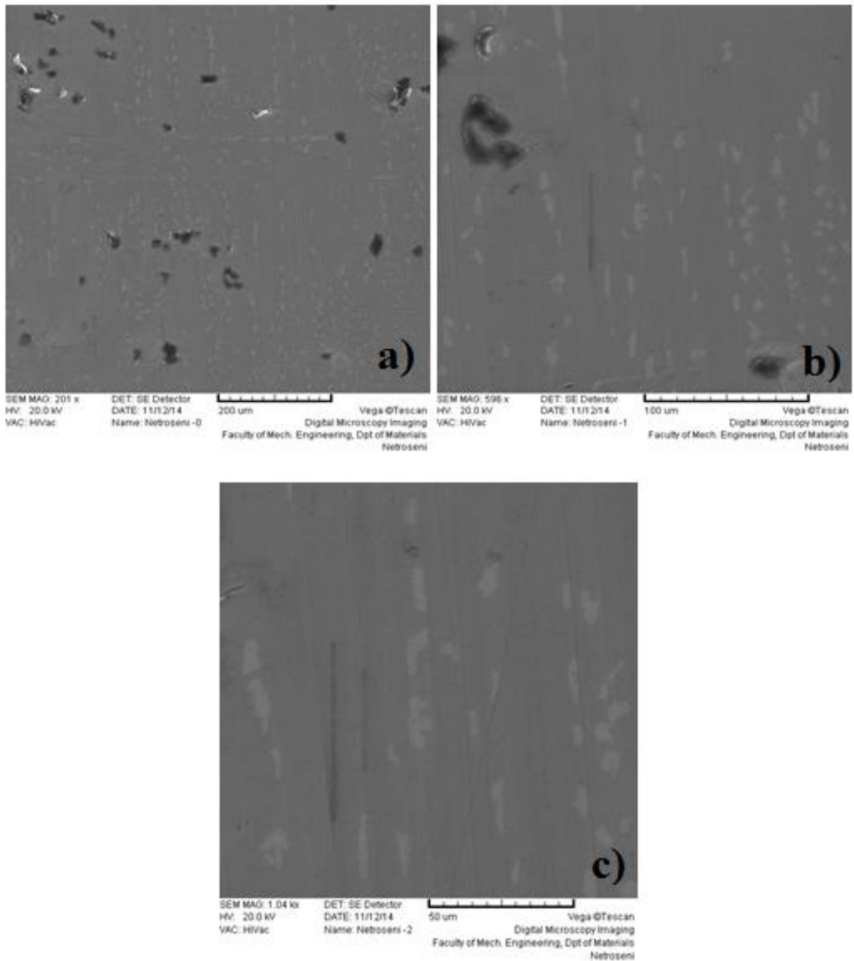
Slika 74. SEM snimka površine netrošenog uzorka (povećanje: a) 200 \mu\text{m} , b) 100 \mu\text{m} , c) 50 \mu\text{m} ).
