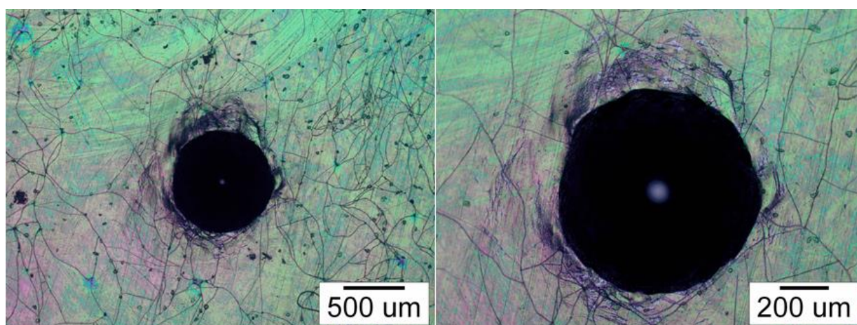
Slika 38. Površina uzorka 2 A (povećanje: lijevo 50x, desno 100x).
