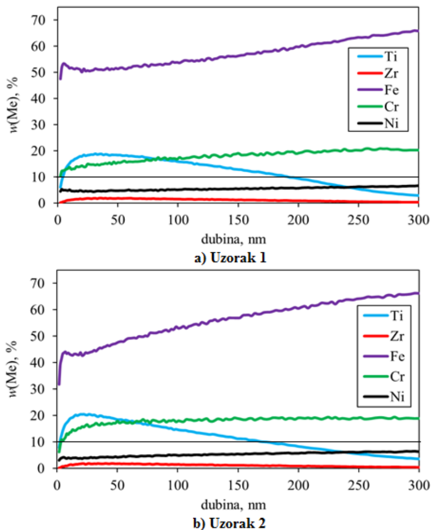
Slika 58. Kvantitativna dubinska profilna analiza uzoraka 1 i 2 (trošeni kvarcni pijeskom, kut 90^\circ , 500 udaraca, Me= Ti, Zr, Fe, Cr, Ni).
