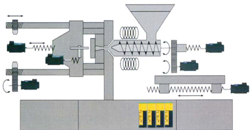
Slika 4.3. Shema električne ubrizgavalice [8]
