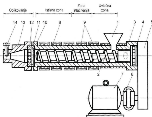
Slika 2.3. Presjek jedнопužnog ekstrudera; 1 – lijevak, 2 – pužni vijak, 3 – cilindar, 4 – tlačni ležaj, 5 – namjestivi prigon, 6 – spojka, 7 – pogonski motor, 8 – grijala, 9 – hladila, 10 – prirubnica, 11 – sita, 12 – cjedilo, 13 – glava ekstrudera, ujedno i mlaznica, 14 – prigušnica [2]
