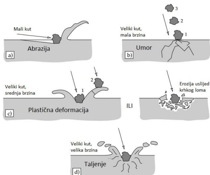
Slika 3. Mogući mehanizmi erozije: a) abrazija pri malim kutevima, b) umor površine pri malim brzinama i velikim kutevima, c) višestruka plastična deformacija ili krhki lom pri srednjim brzinama i velikim kutevima, d) taljenje površine uslijed velikih brzina udara [3]
