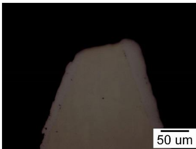
Slika 11. Detaljniji prikaz bočnog presjeka vrha zuba u poliranom stanju.
