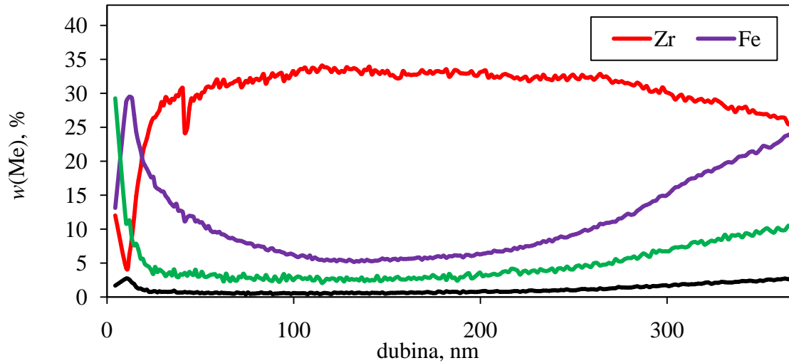
Slika 36. Kvantitativna dubinska profilna analiza (GDS-QDP) sol-gel \text{ZrO}_2 filmova na nehrđajućem čeliku, ovisnost atomskih udjela pojedinih elemenata (%) o dubini (nm) kod uzorka 2D-GORE ( \vartheta_k = 400 \text{ }^\circ\text{C} , \alpha = 30^\circ , 500 udaraca)
