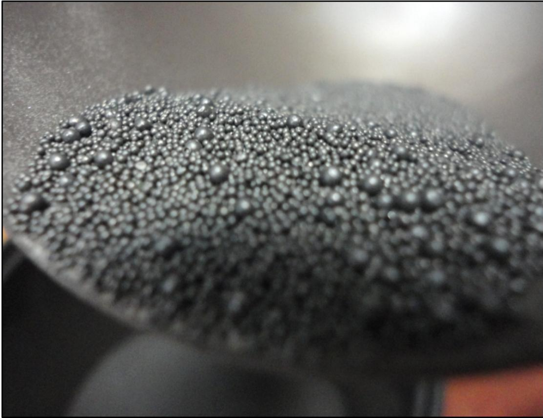
Slika 14. Prikaz čelične sačme promjera ~700 \mu\text{m}
