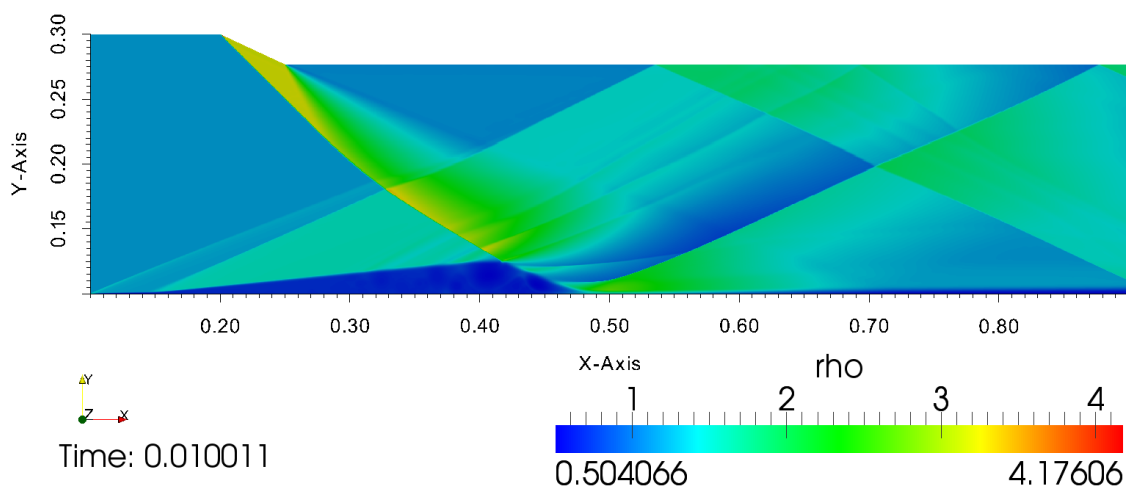
Slika 4.37: Polje gustoće izraženo \text{kg}/\text{m}^3 za najfiniju mrežu.
