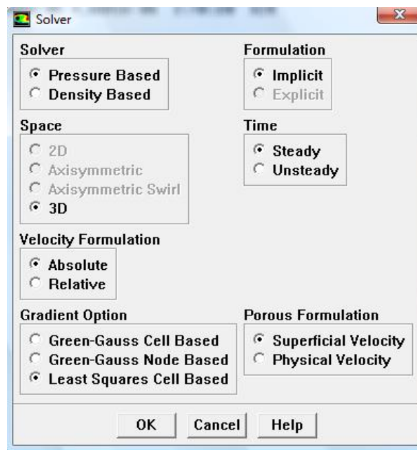
Slika 3.12. Definiranje solvera
