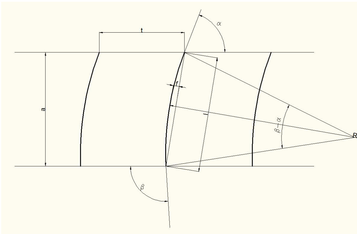
Slika 2.11. Geometrija kružnog isječka
