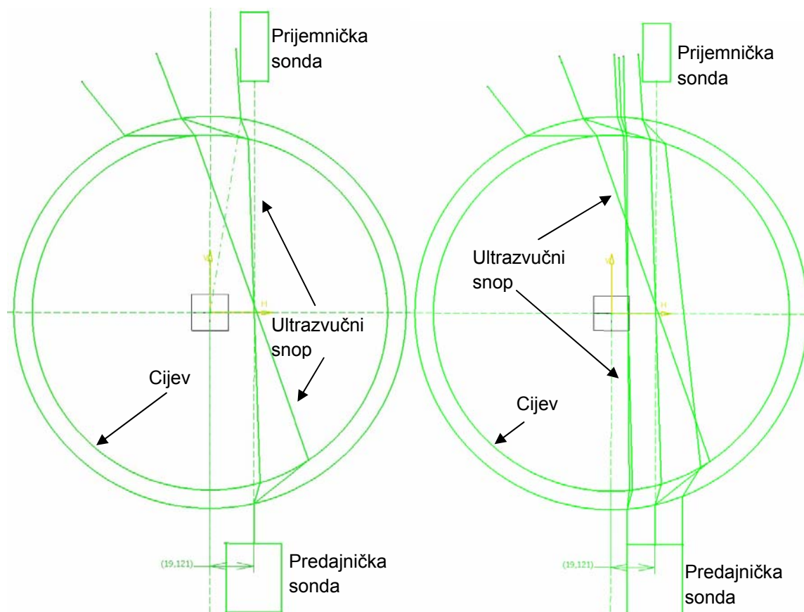
Slika 34. Položaj sonde 7
