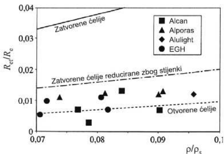
Slika 3.4. Ovisnost omjera granice stlačivanja pjene ( R_{et} ) i granice tečenja materijala ćelija ( R_e ) o relativnoj gustoći /14/
