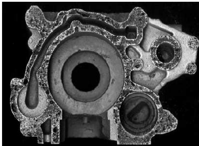
Slika 5.11. Lijevani proizvod od aluminijске pjene /26/
