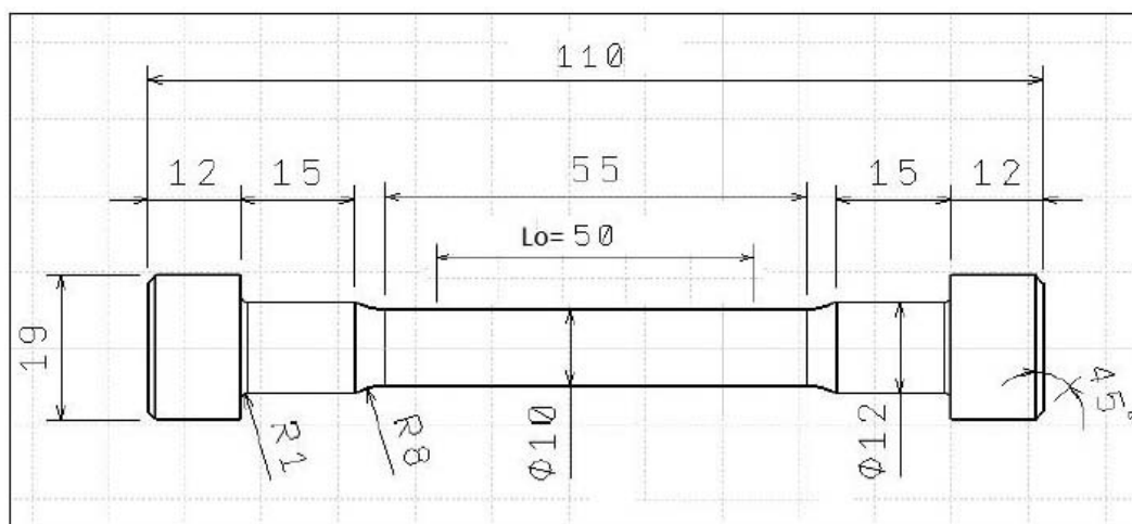
Slika 48. Dimenzije epruvete
