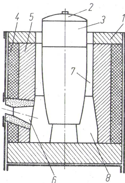
Slika 11. Peć s loncem [11]: 1 poklopac peći, 2 poklopac lonca, 3 nastavak, 4 izolacija, 5 obloga, 6 plamenik, 7 ogrjevna komora, 8 komora za izgaranje
