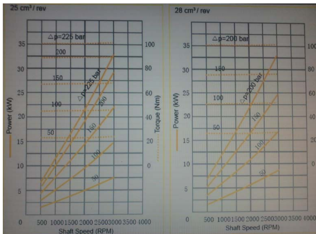
Slika 8. Snaga potrebna za pokretanje pumpe grupe 2
