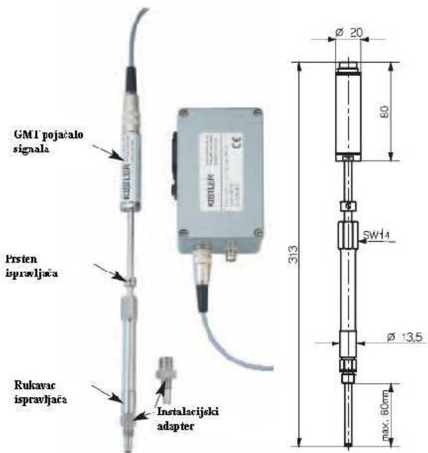
Slika 11. Struktura sustava GMT senzora
