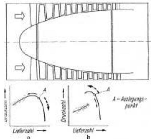
Abb. 501 a u. b. Abreiß-Charakteristik einer Eintrittsstufe (a) und einer Endstufe (b) eines mehrstufigen Axialverdichters
