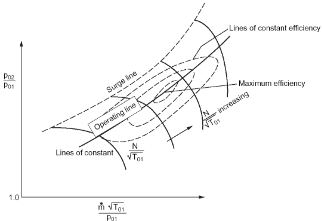
slika 4.1 tipična karta performansi dobivena testiranjem kompresora
