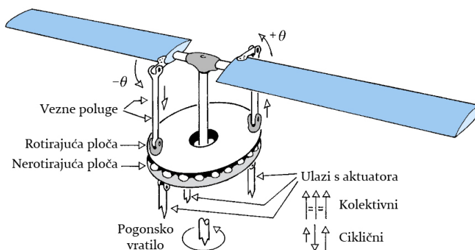
Slika 2.9: Zakretna ploča [3]
