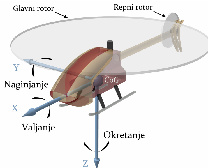
Slika 2.4: Helikopter
