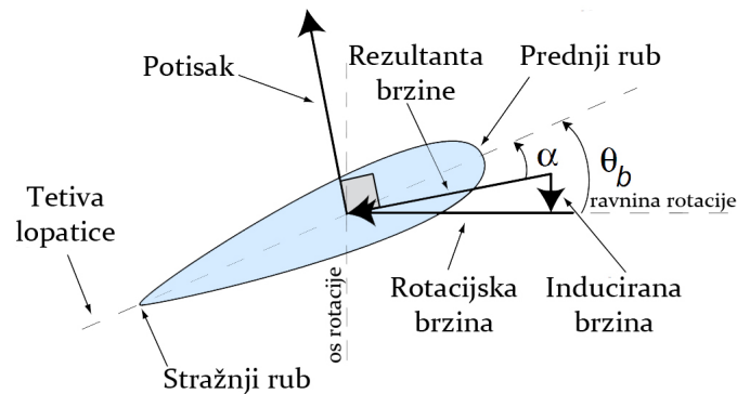
Slika 2.5: Prikaz sila na lopatici rotora [3]
