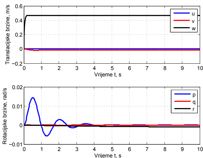
Slika 5.8: Odziv nelinearnog modela helikoptera s LQ regulatorom
