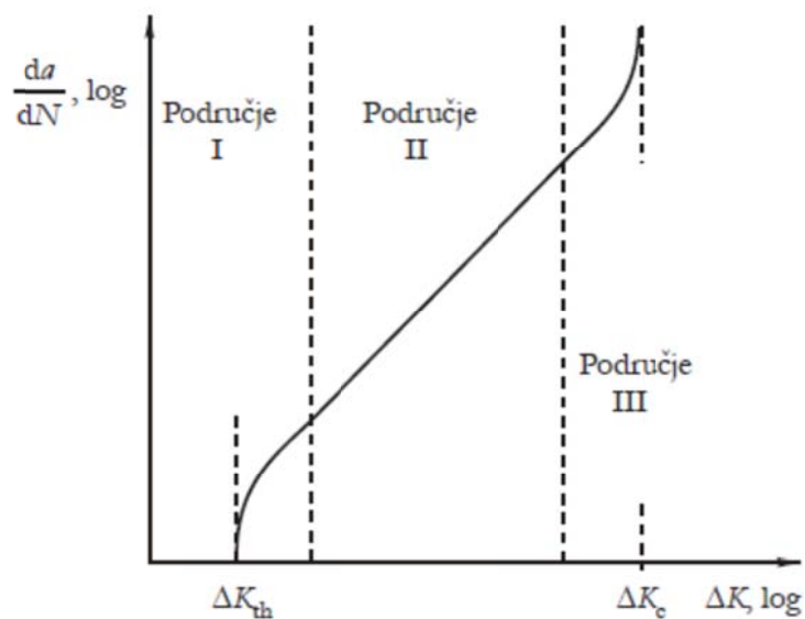
Slika 17. Tipična krivulja relativnog rasta pukotine
