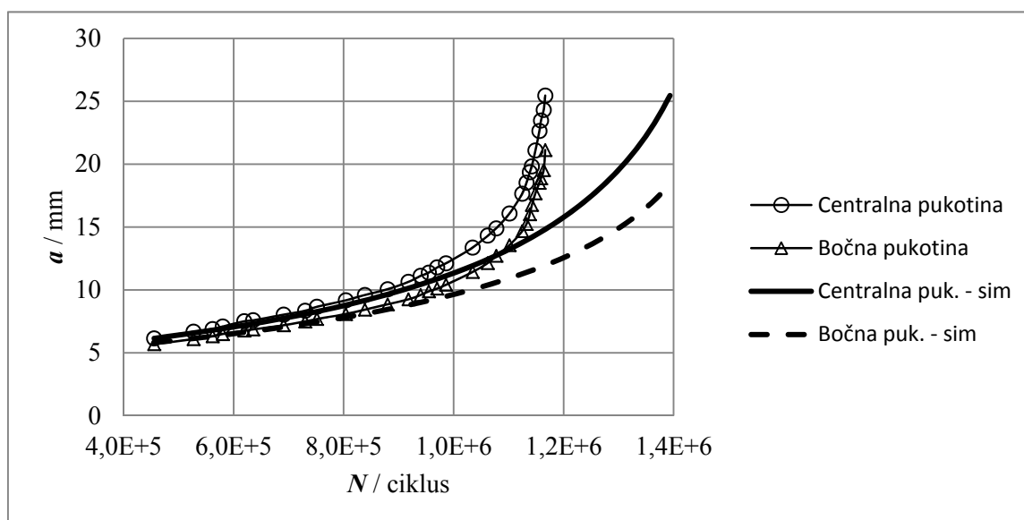
Slika 65. Usporedba eksperimentalnog i simuliranog životnog vijeka (Paris, P3)
