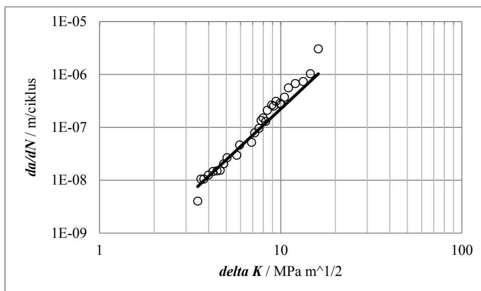
Slika 57. Dijagram relativnog napredovanja pukotine (Forman, P1)
