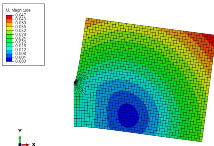
Slika 32. Prikaz kontura pomaka (fina mreža)
