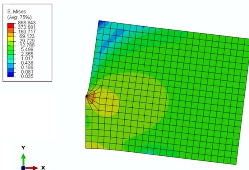
Slika 31. Prikaz kontura napreznja (srednja mreža)
