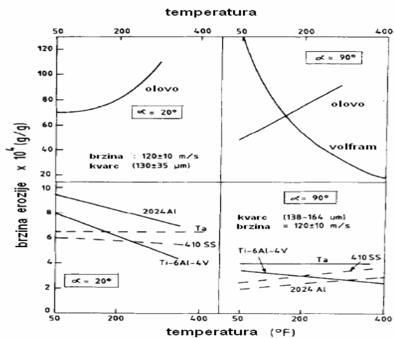
Slika 25. Ovisnost brzine erozije o temperaturi za neke materijale pri različitim kutovima udara, [4]
