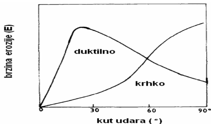
Slika 13. Brzina erozije u funkciji kuta udara čestica za duktilne i krhke materijala [4]
