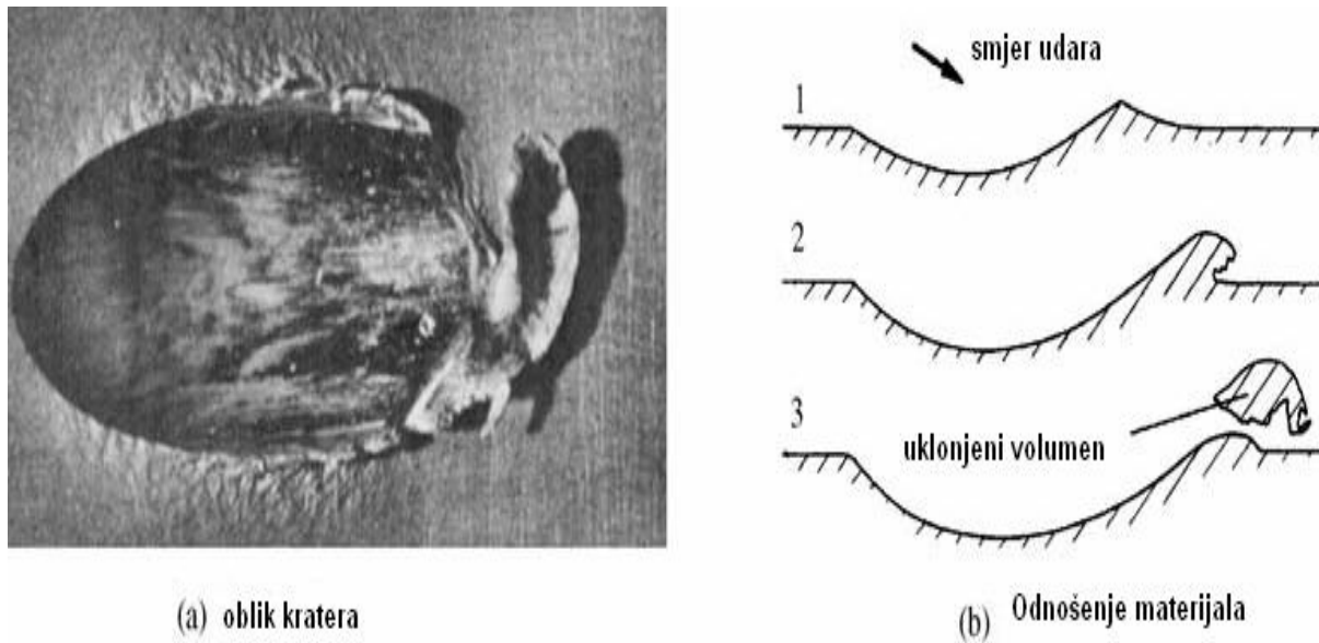
Slika 16. Oblik kratera i mehanizam odnošenja kod duktilnih materijala [4]
