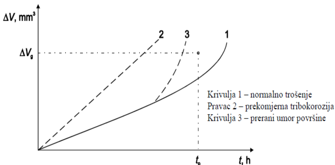
Slika 46. Procesi trošenja pri kavitacijskoj eroziji [4]
