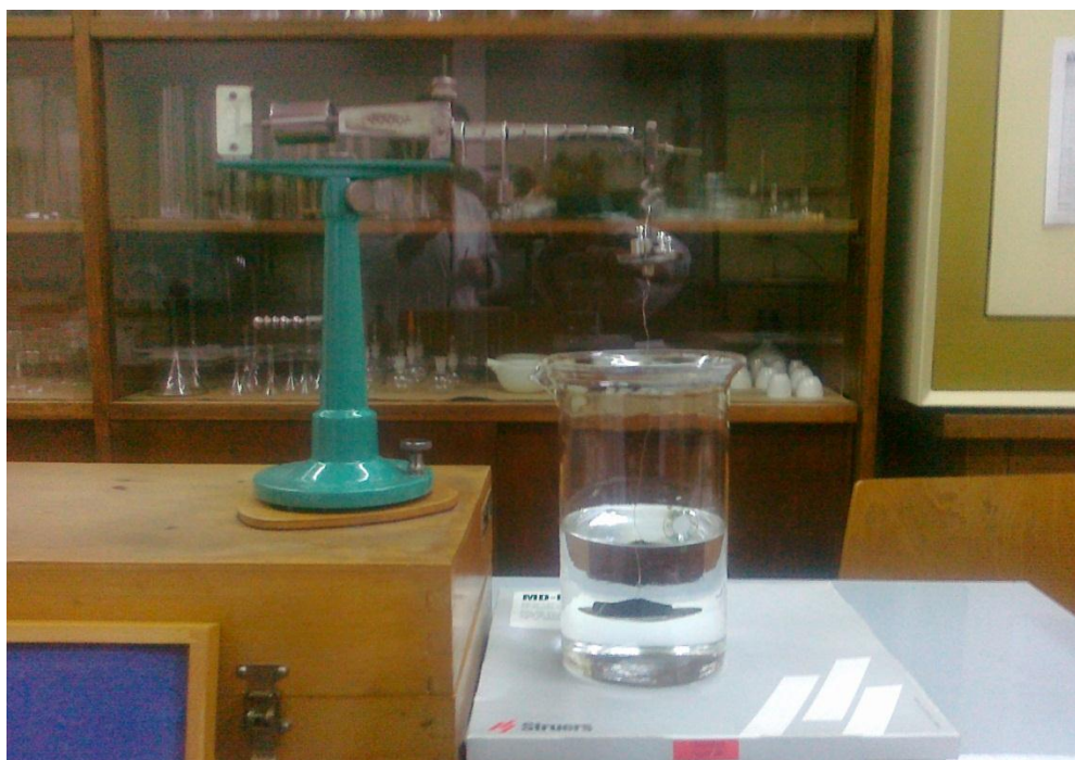
Slika 80. Vaga i hidrostatsko mjerenje uzoraka 1 i 2
