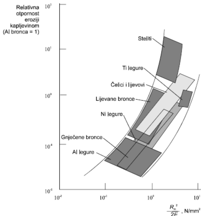
Slika 36. Relativna otpornost nekih materijala na eroziju kapljevinaom, [4]
