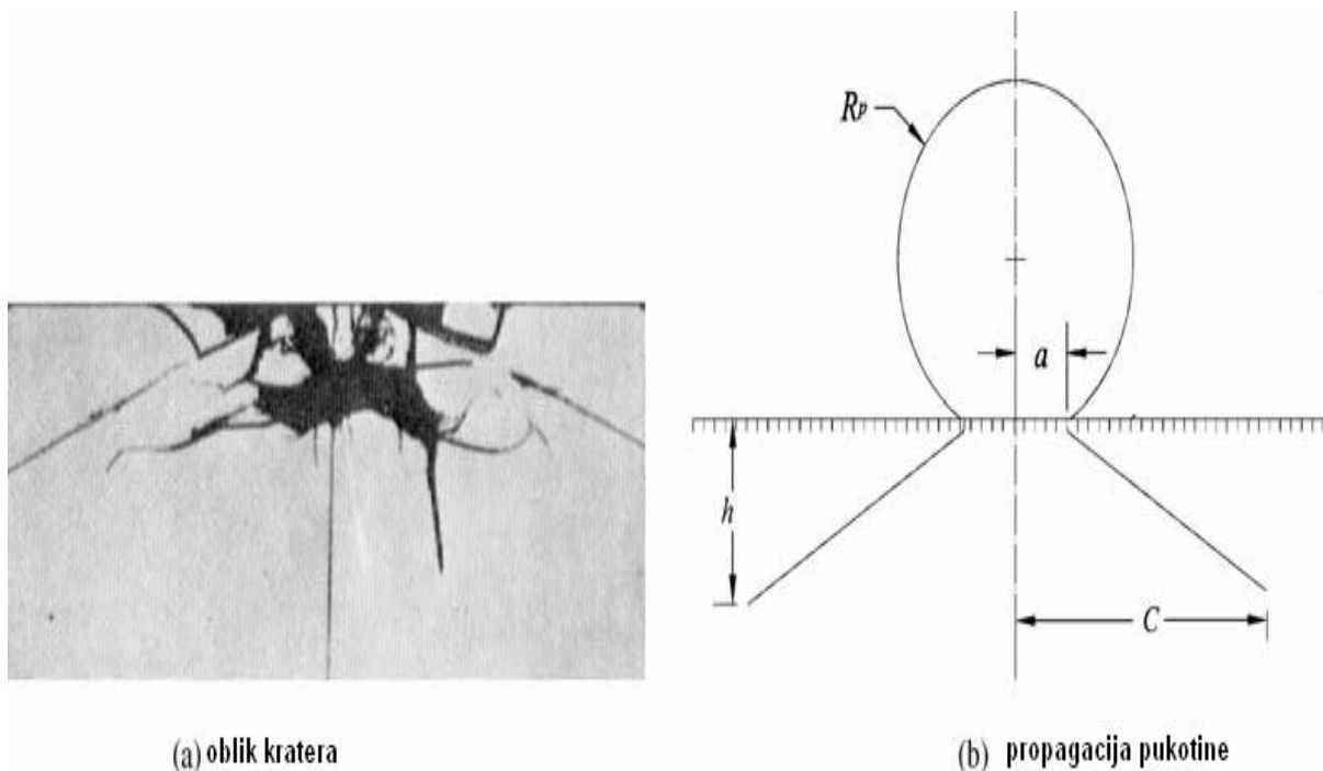
Slika 17. Oblik kratera i mehanizam propagacije pukotine kod krhkih materijala [4]
