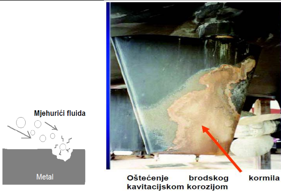
Slika 7. Kavitacijska korozija [5]
