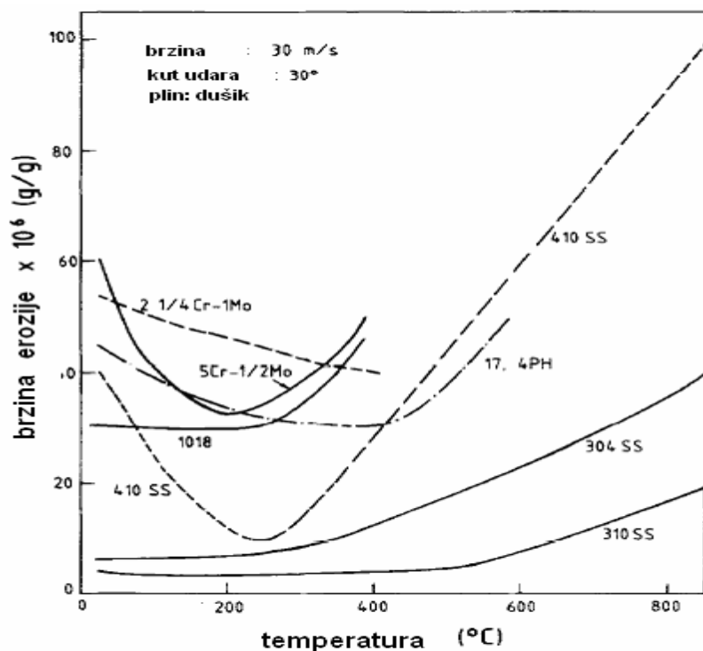
Slika 24. Ovisnost brzine erozije o temperaturi za neke materijale, [4]
