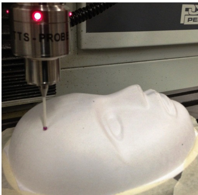
Slika 22. Kontaktni skener
