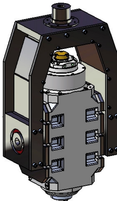
Slika 83. Motorvretno sa konstrukcijom okretno nagibne glave
