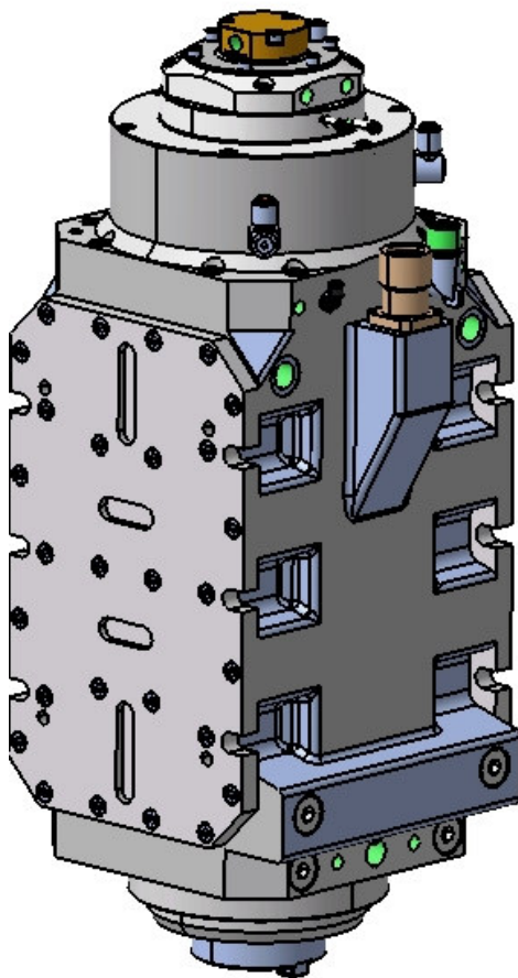
Slika 57. Motorvreteno VA14 [12]
