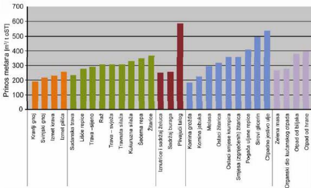
Slika 6. Prinos metana po vrsti sirovine
