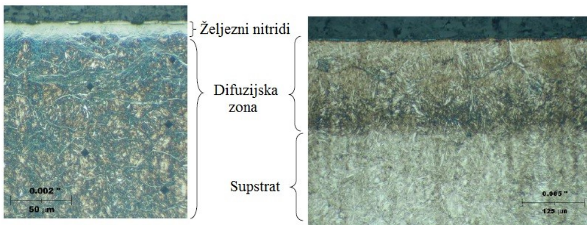
Slika 12. Mikrostruktura legure za nitiranje komercijalnog naziva Nitralloy 135M nakon kaljenja i popuštanja te plinskog nitiranja [3]
