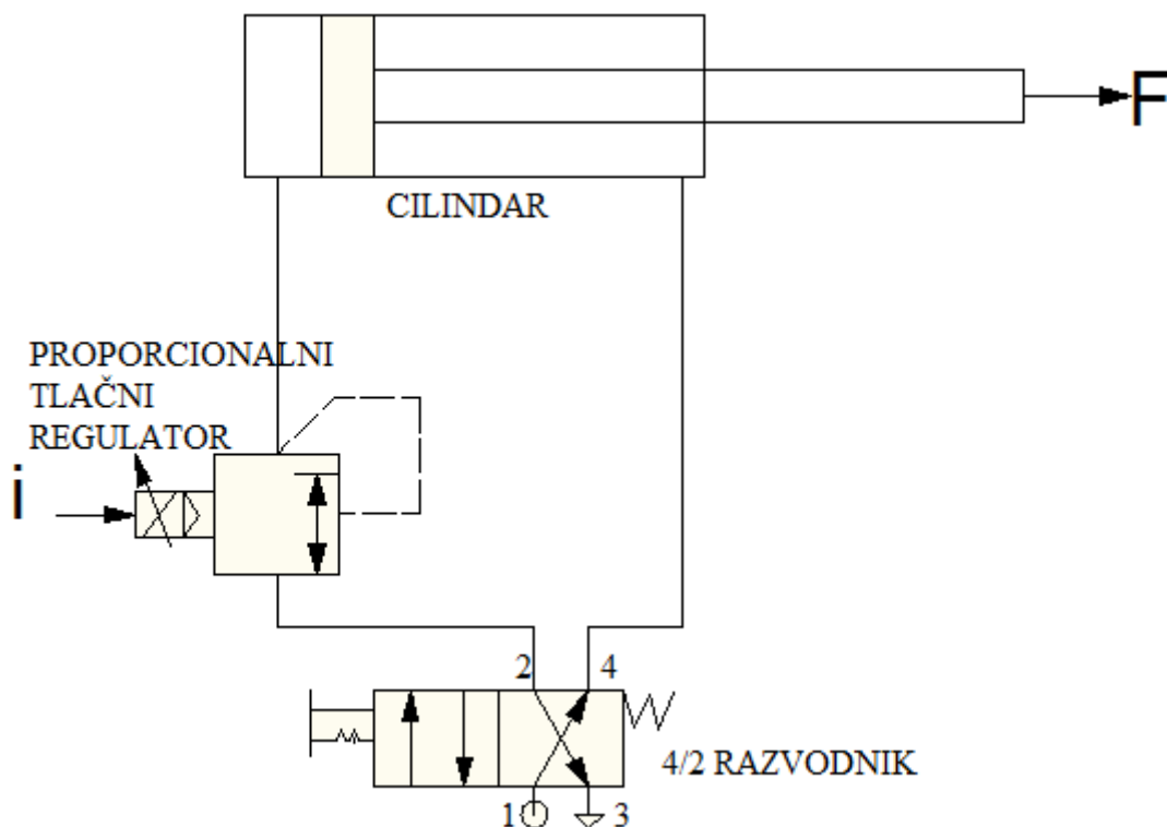
Slika 31 Shema spajanja
