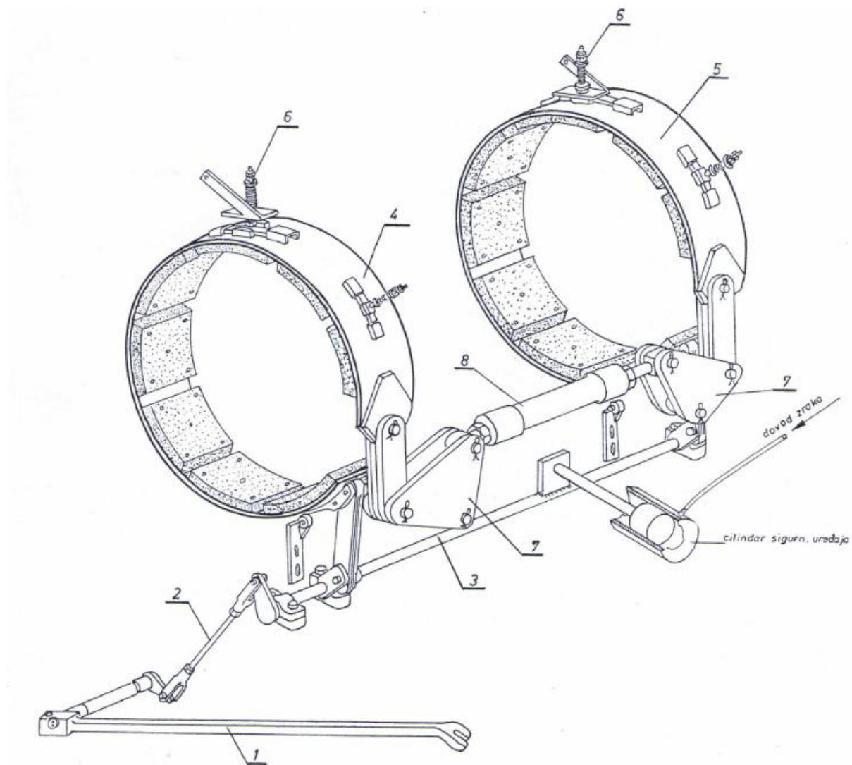
Slika 14 Pojasna kočnica Cardwell [5]
