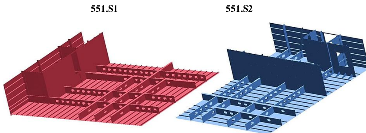
Slika 5. Sekcije palube 8
