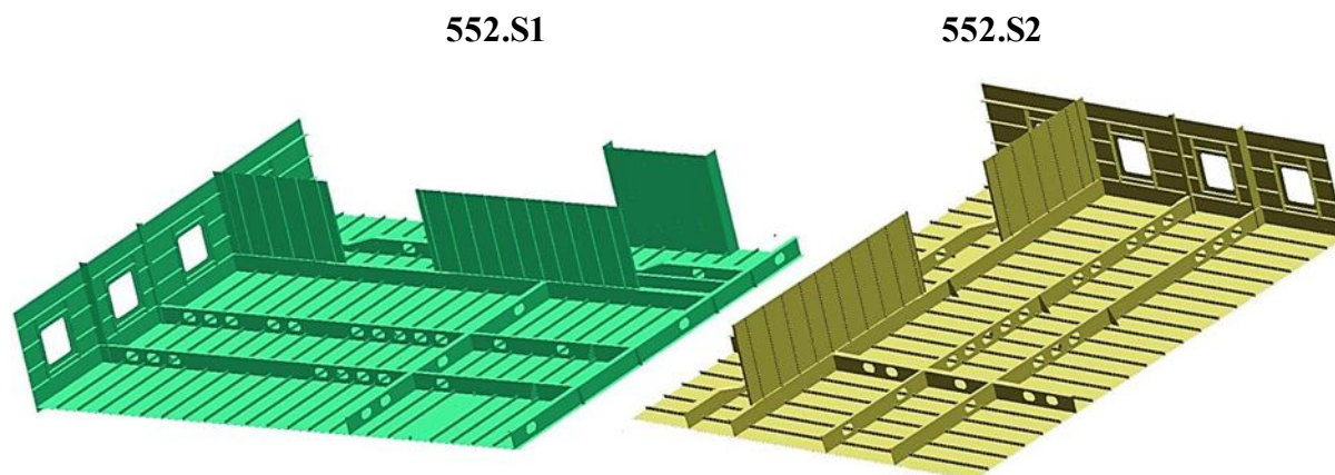
Slika 6. Sekcije palube 9
