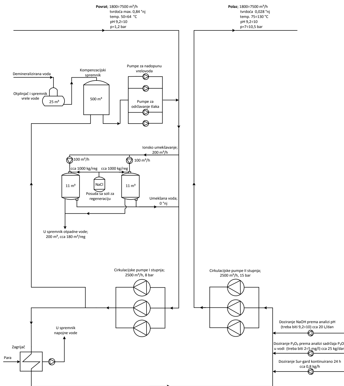
Slika 4. Pojednostavljena shema vrelvodnog sustava TE-TO Zagreb
