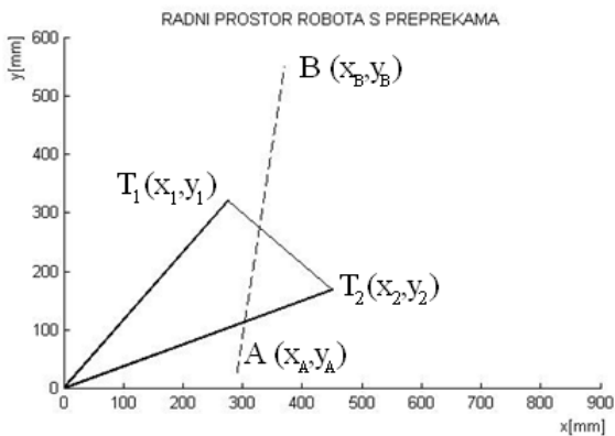
Slika 3.25 Granični uvjet 9
