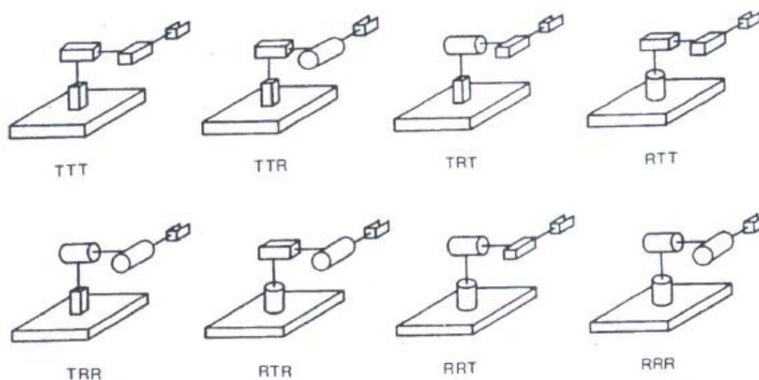
Slika 2.5 Kinematičke strukture robota
