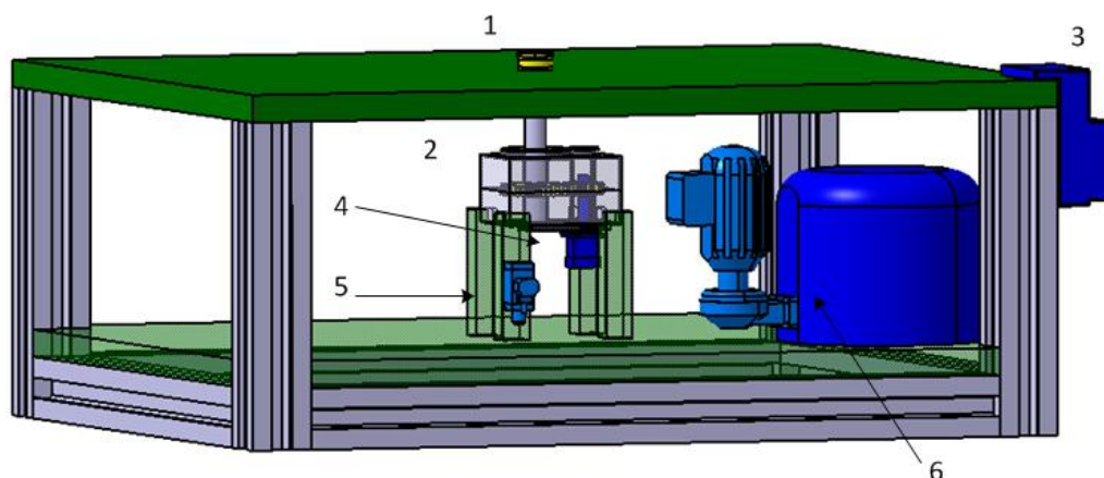
Slika 5.7 Pogonski dio sustava robota
