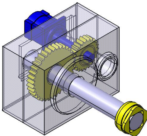
Slika 5.2 Projektirani reduktor
