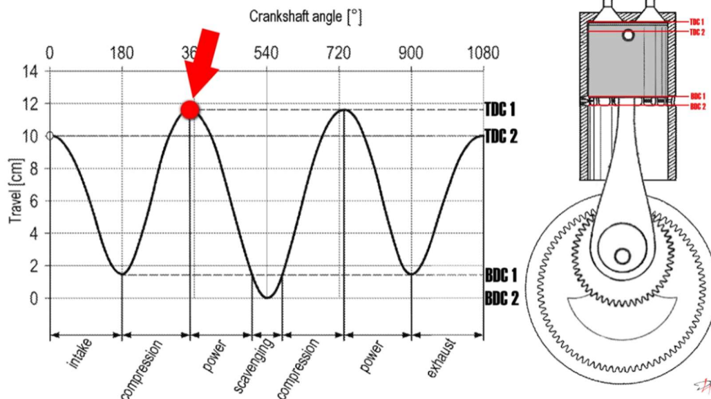
Slika 19. Kompresijski takt na kraju [3]
