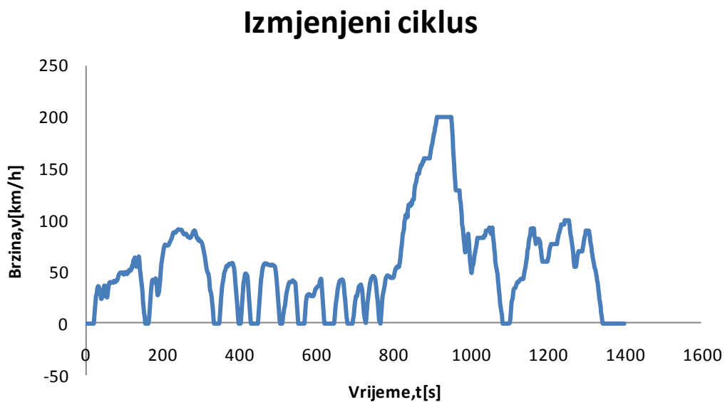
Slika 4.3.-Izmjenjeni ciklus
