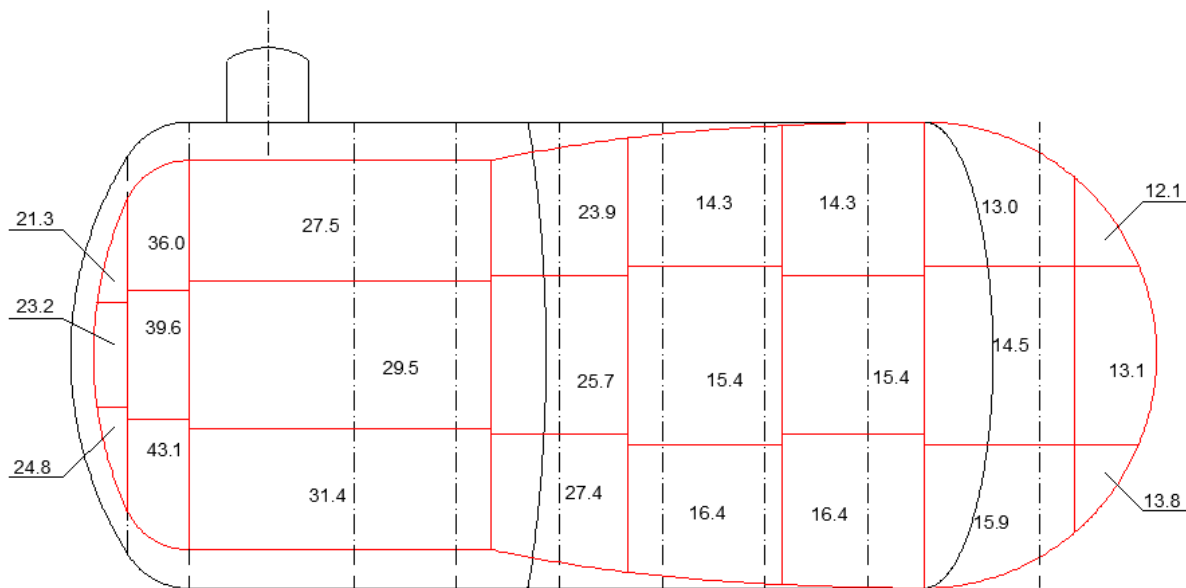
Slika 5.1. Debljine stijenke uzdužne pregrade
