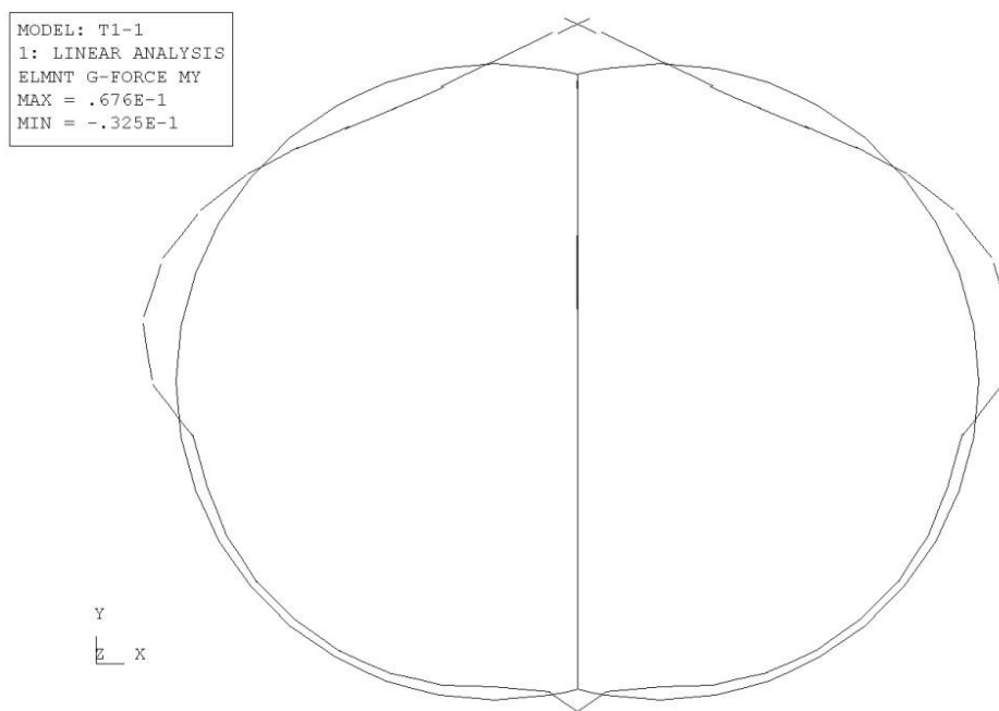
Slika 6.21. Moment savijanja M_y za SR2
