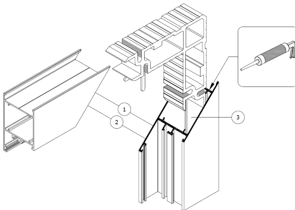
Slika 26. Spajanje profila kutnicima pod kutem od 90° [16]
