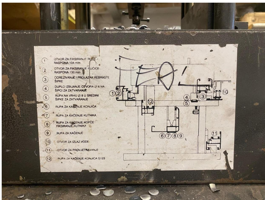
Slika 23. Popis i prikaz namjena štancanja na štanci
