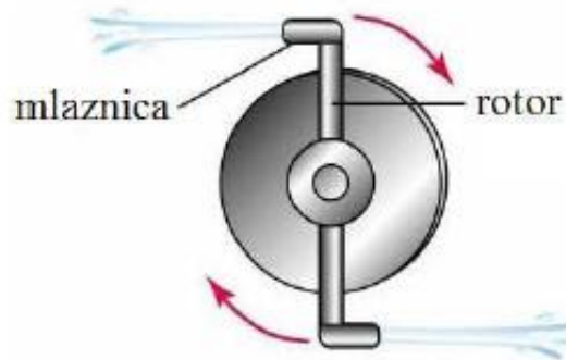
Slika 5. Reakcijska turbina
