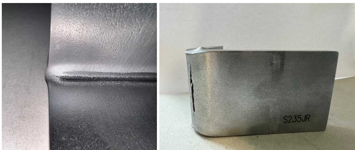
Slika 48. Rubna izobličenja i ostale greške na S235JR
