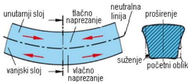
Slika 12. Kutno savijanje lima [12]
