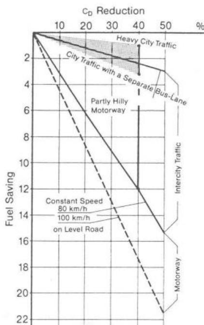
Slika 3. Ovisnost faktora otpora zraka o uštedi goriva[2]
