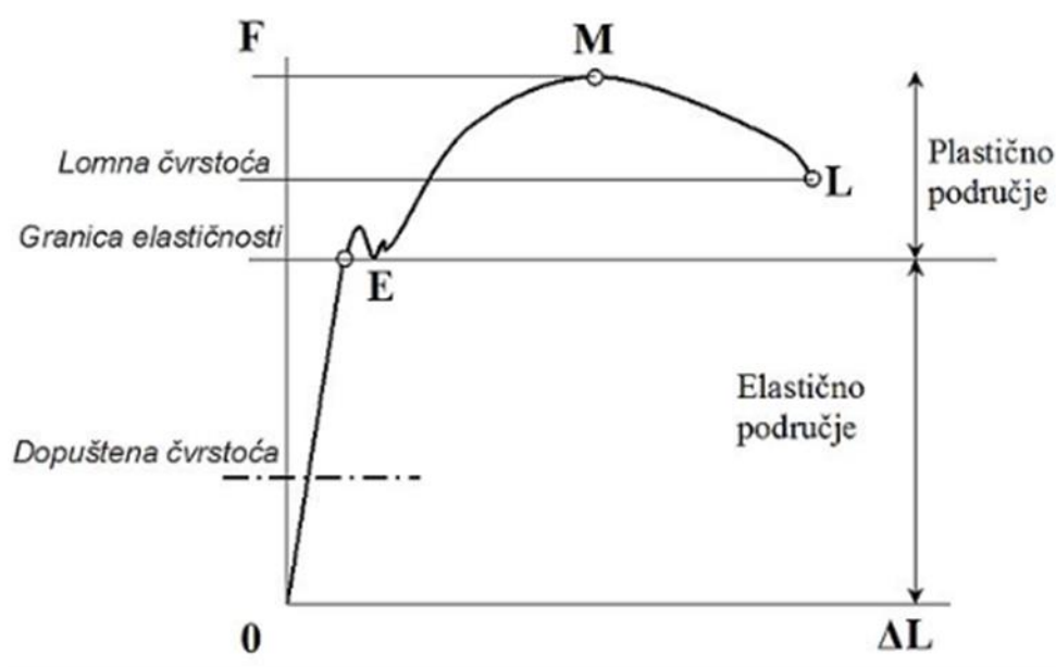
Slika 6. Dijagram naprezanja-Hookov zakon
