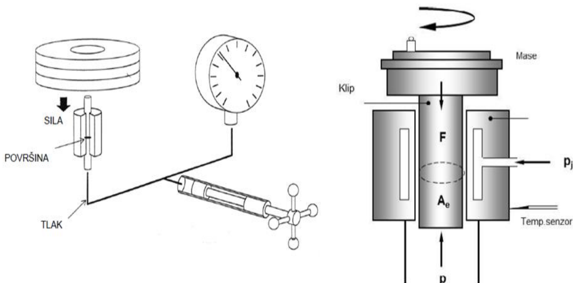
Slika 4. Sklop klipa i cilindra na tlačnoj vagi
