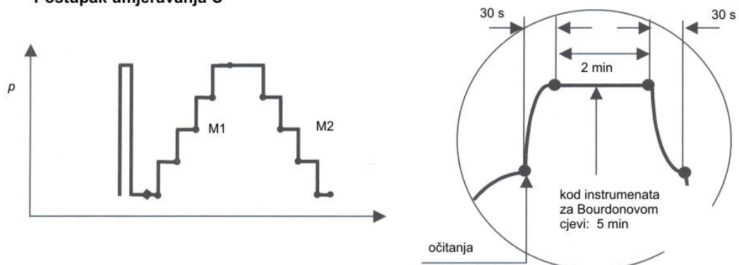
Slika 5. Postupci umjeravanja
