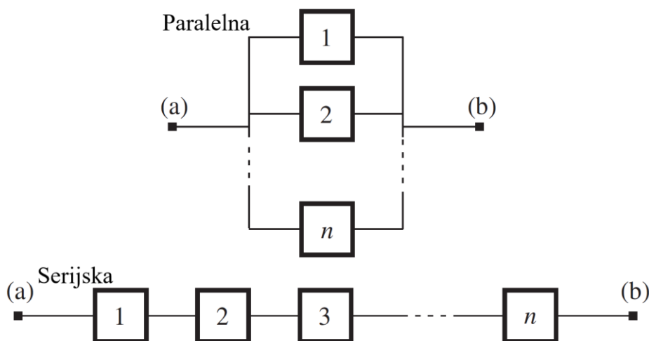
Slika 2. Konfiguracije sustava [21]
