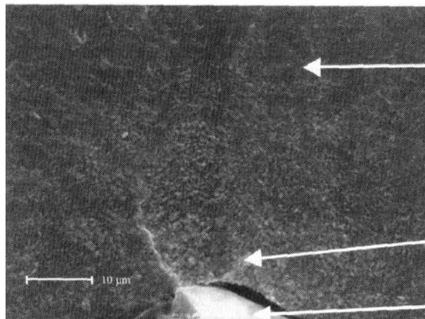
Slika 20. Tvrda uključina kao izvor ispod površinskog začea pukotine Cr-Mo čelika
