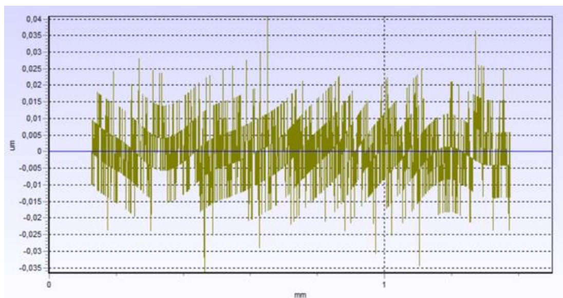
Slika 30. Profil hrapavosti površine prstena B2
