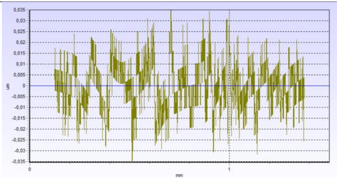
Slika 29. Profil hrapavosti površine prstena B1
