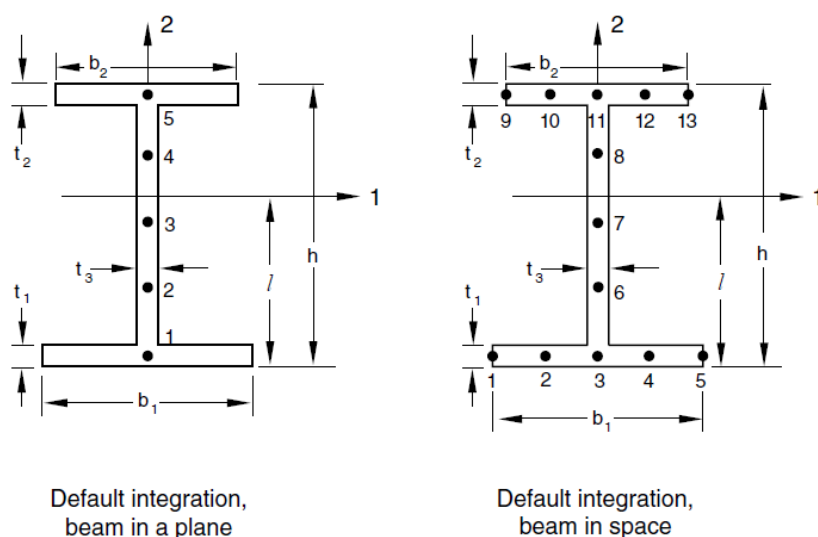
Slika 6. Poprečni presjek I-profila [3]
