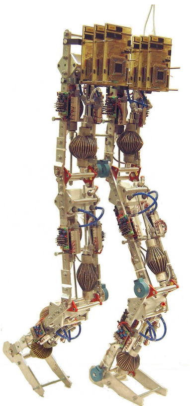
Slika 2.14. Hodajući robot „Lucy“ [13]
