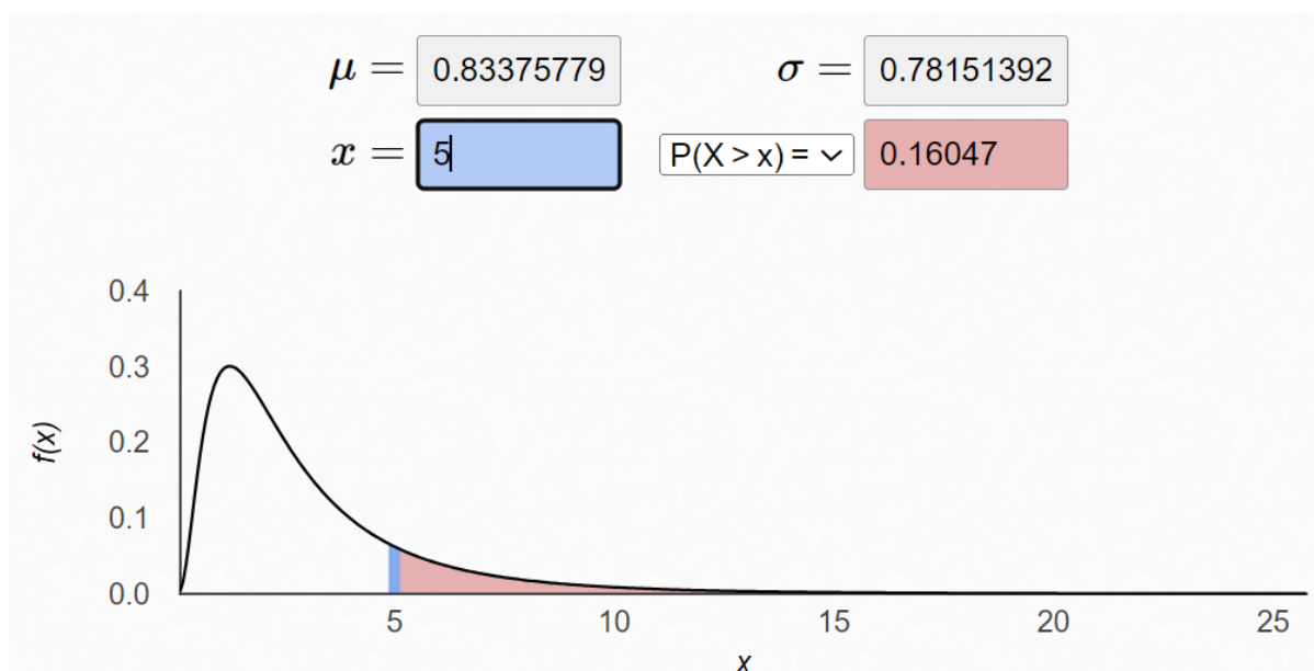
Slika 24. Grafički prikaz udjela dodatnog trafo lima koji prelazi 5% na stroju 4
