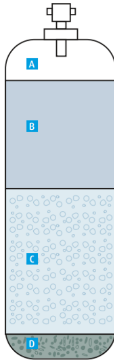
Slika 22. Shema boce za acetylen [41]
